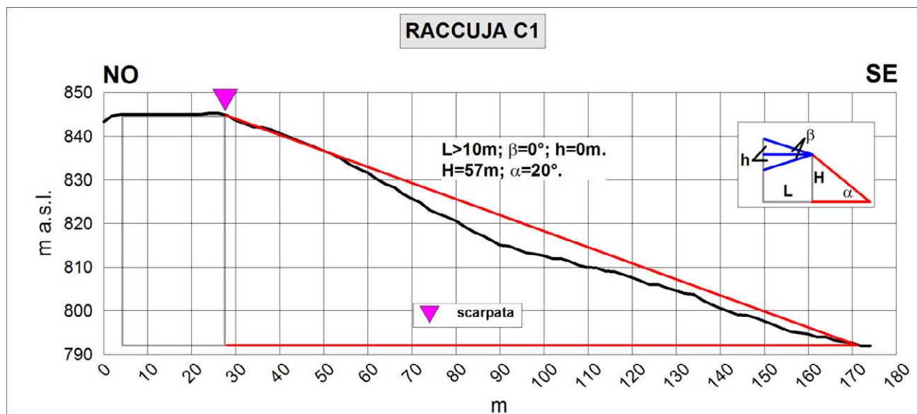
Fig. 8.16 – Profilo topografico di dettaglio della scarpata Raccuja C1.
