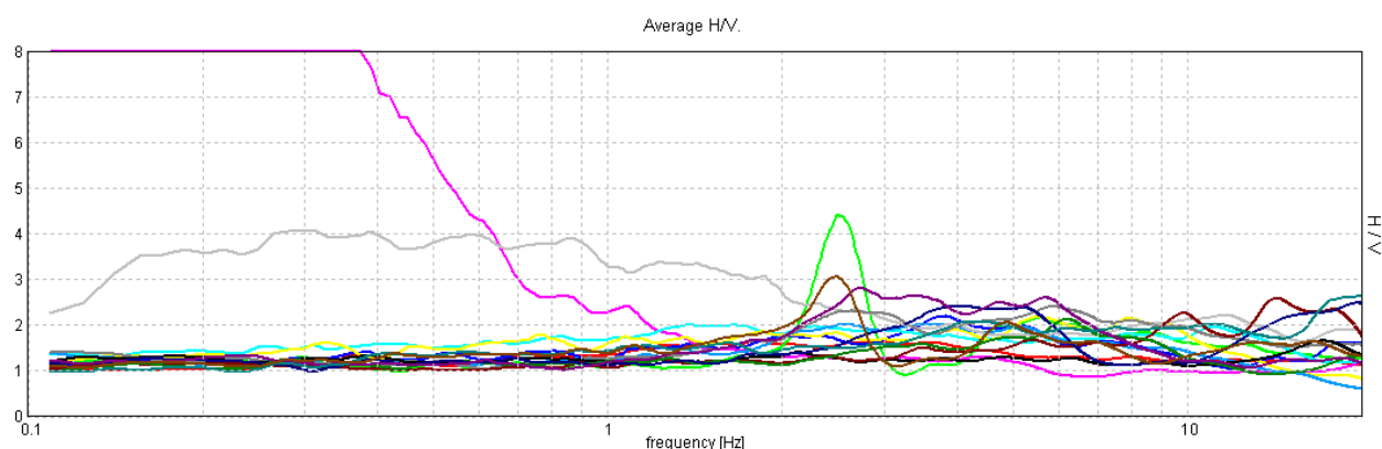
Fig. 4.5 – Segnali HVSR registrati dalle 16 stazioni singole.
