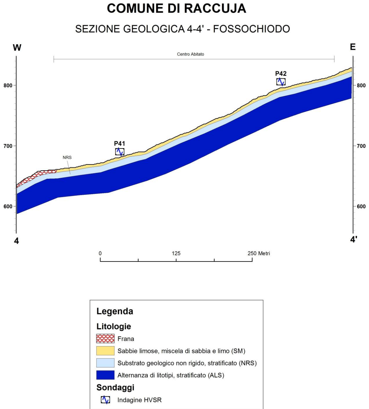
Fig. 5.4 – Sezione geologica W – E attraverso l’abitato di Fossochiodo (per l’ubicazione si veda la Carta Geologico – tecnica).
