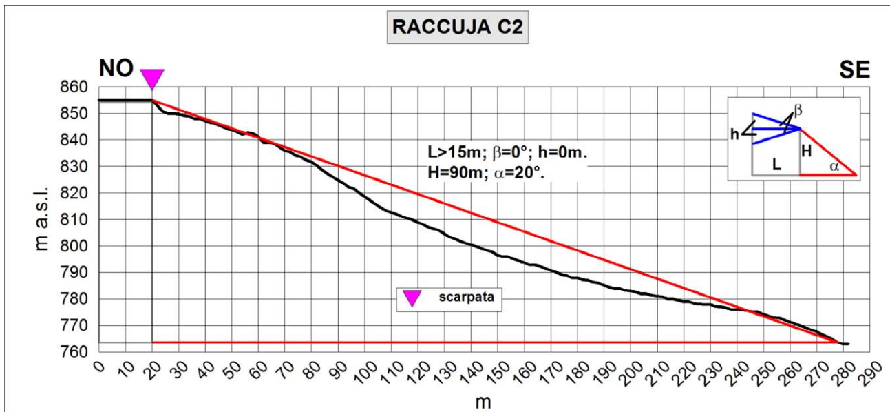
Fig. 8.17 – Profilo topografico di dettaglio della scarpata Raccuja C2.
