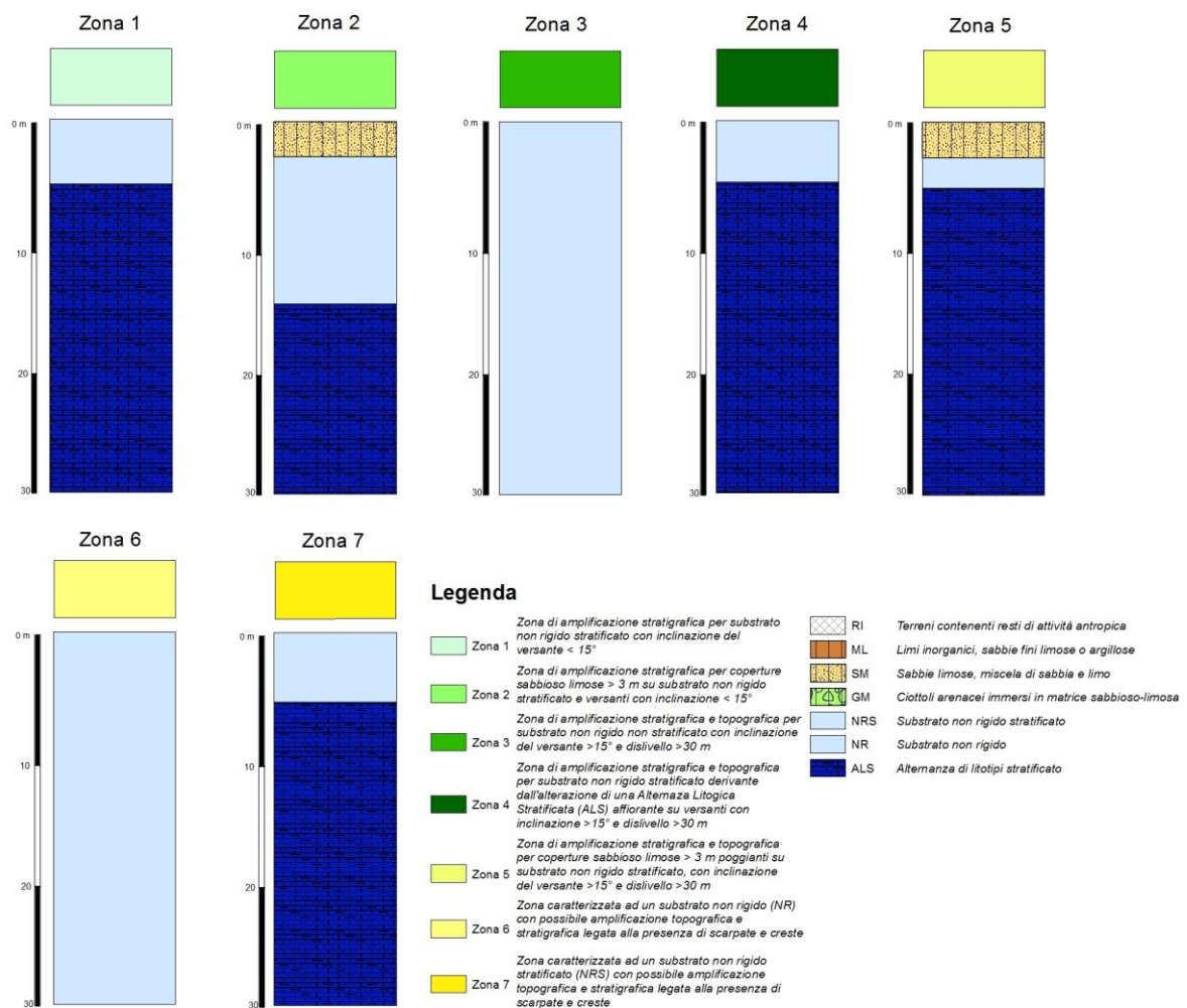
Fig. 8.4 – Colonne rappresentative delle zone suscettibili di amplificazione sismica.
