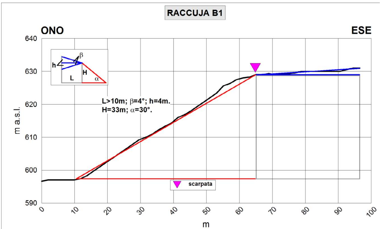
Fig. 8.13 – Profilo topografico di dettaglio della scarpata Raccuja B1.
