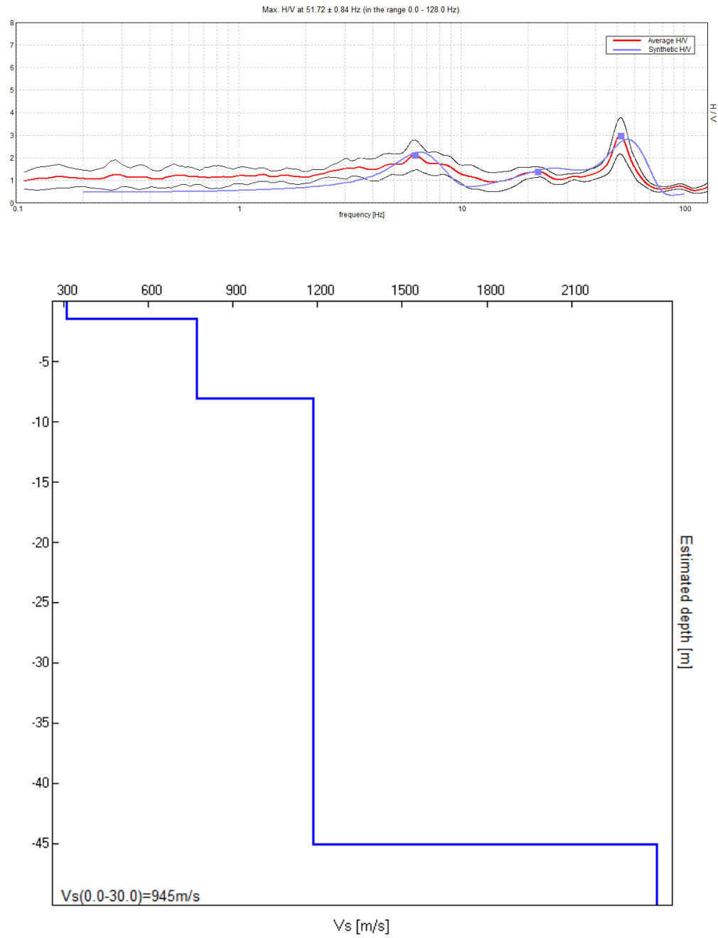
Fig. 5.6 – Esempio di modello monodimensionale a strati della velocità delle onde di taglio ottenuta dall'inversione del sondaggio 83069P32-HVSR105.
