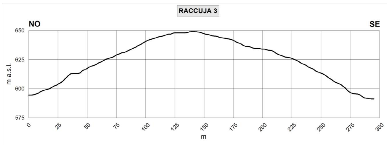
Fig. 3.8c – Profilo topografico di inquadramento Raccuja 3.
