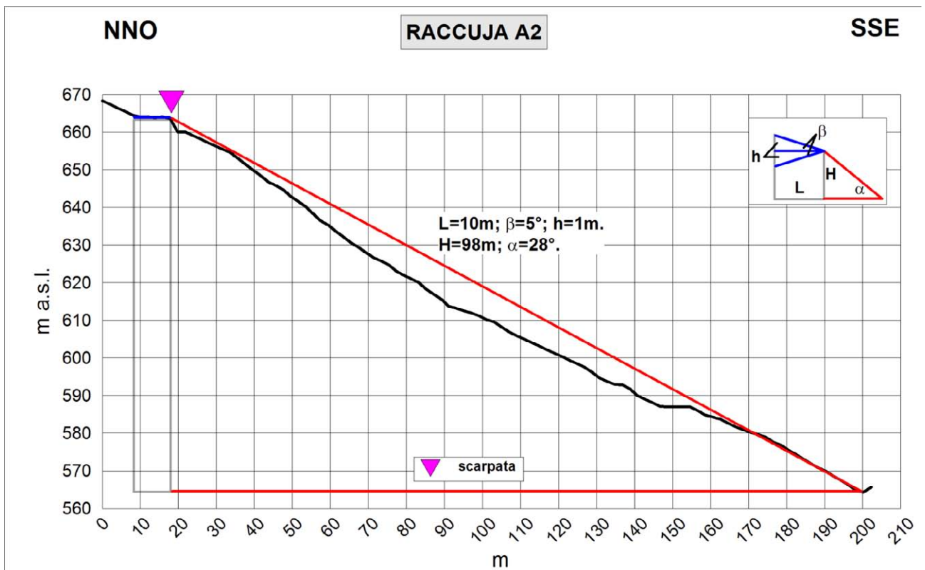
Fig. 8.10 – Profilo topografico di dettaglio della scarpata Raccuja A2.
