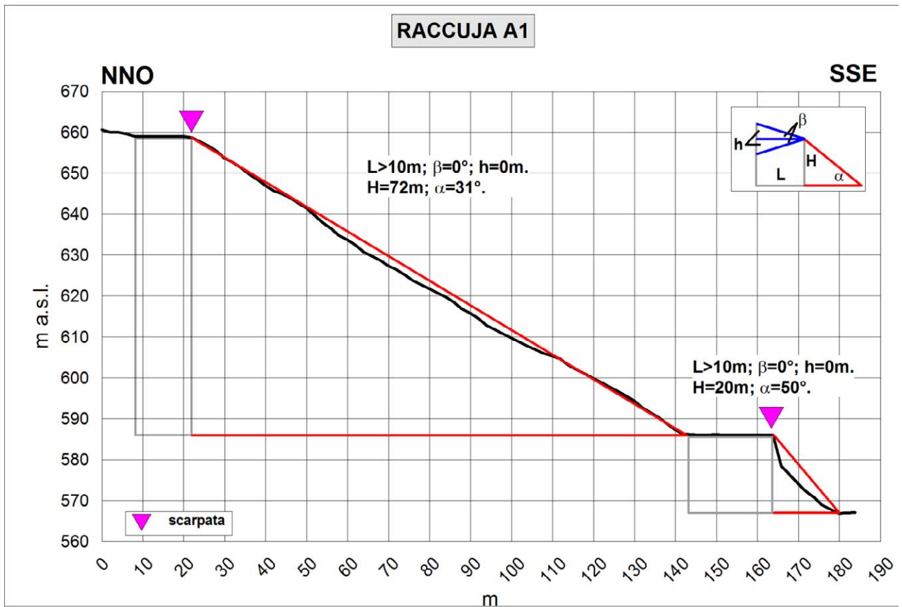
Fig. 8.9 – Profilo topografico di dettaglio della scarpata Raccuja A1.
