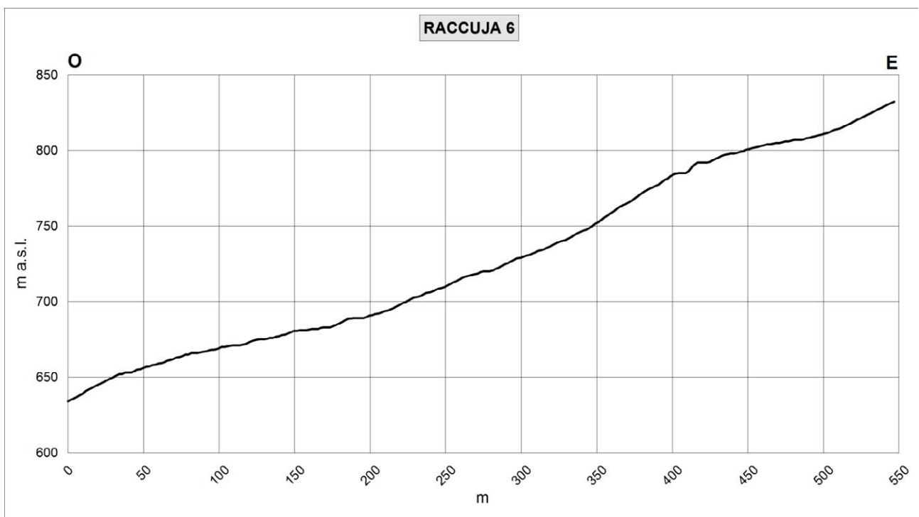
Fig. 3.8f – Profilo topografico di inquadramento Raccuja 6 (Fossochiodo).
