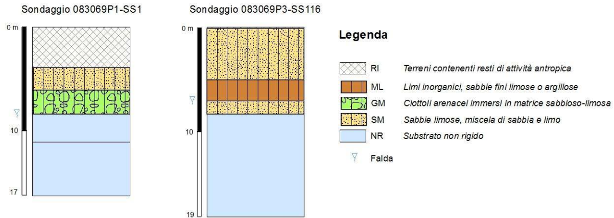
Fig. 5.5 – Sondaggi rappresentativo del sottosuolo del settore settentrionale dell'area perimetrata del centro urbano principale di Racuja
