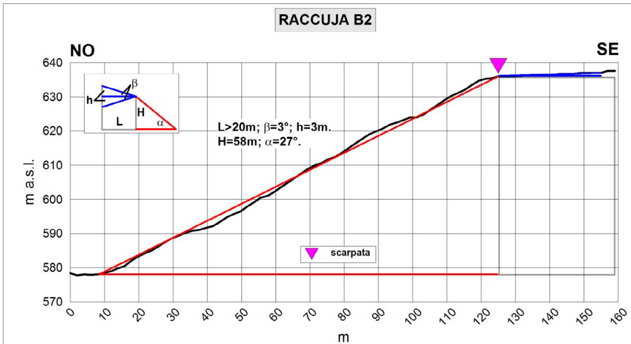
Fig. 8.14 – Profilo topografico di dettaglio della scarpata Raccuja B2.
