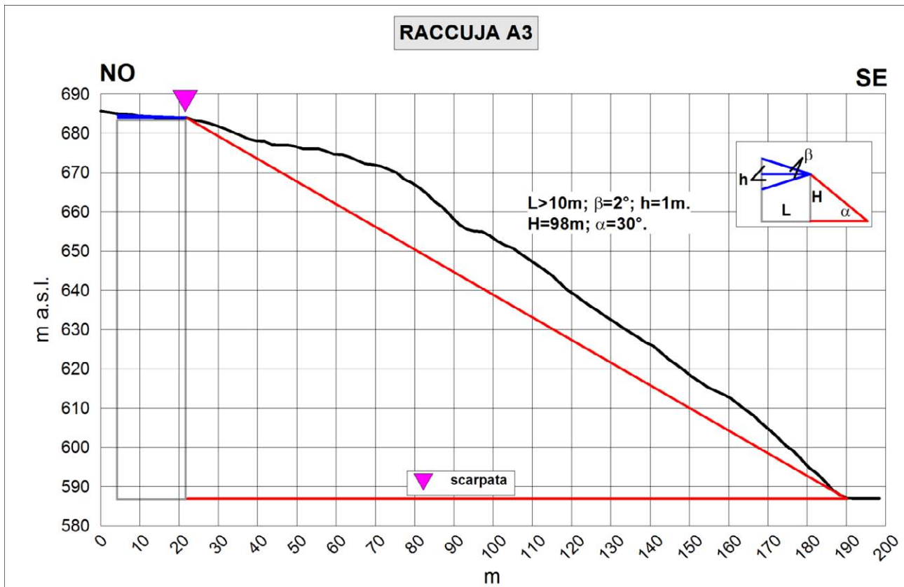
Fig. 8.11 – Profilo topografico di dettaglio della scarpata Raccuja A3
