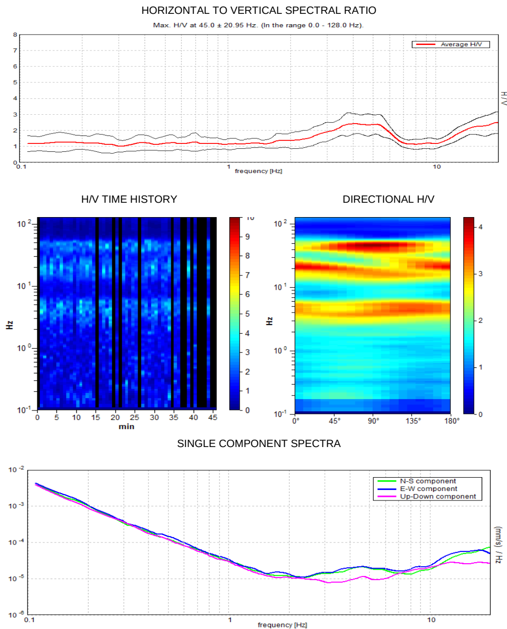
Fig. 4.4 – Analisi dei dati relativi al punto di misura 083069P41-HVSR119.
