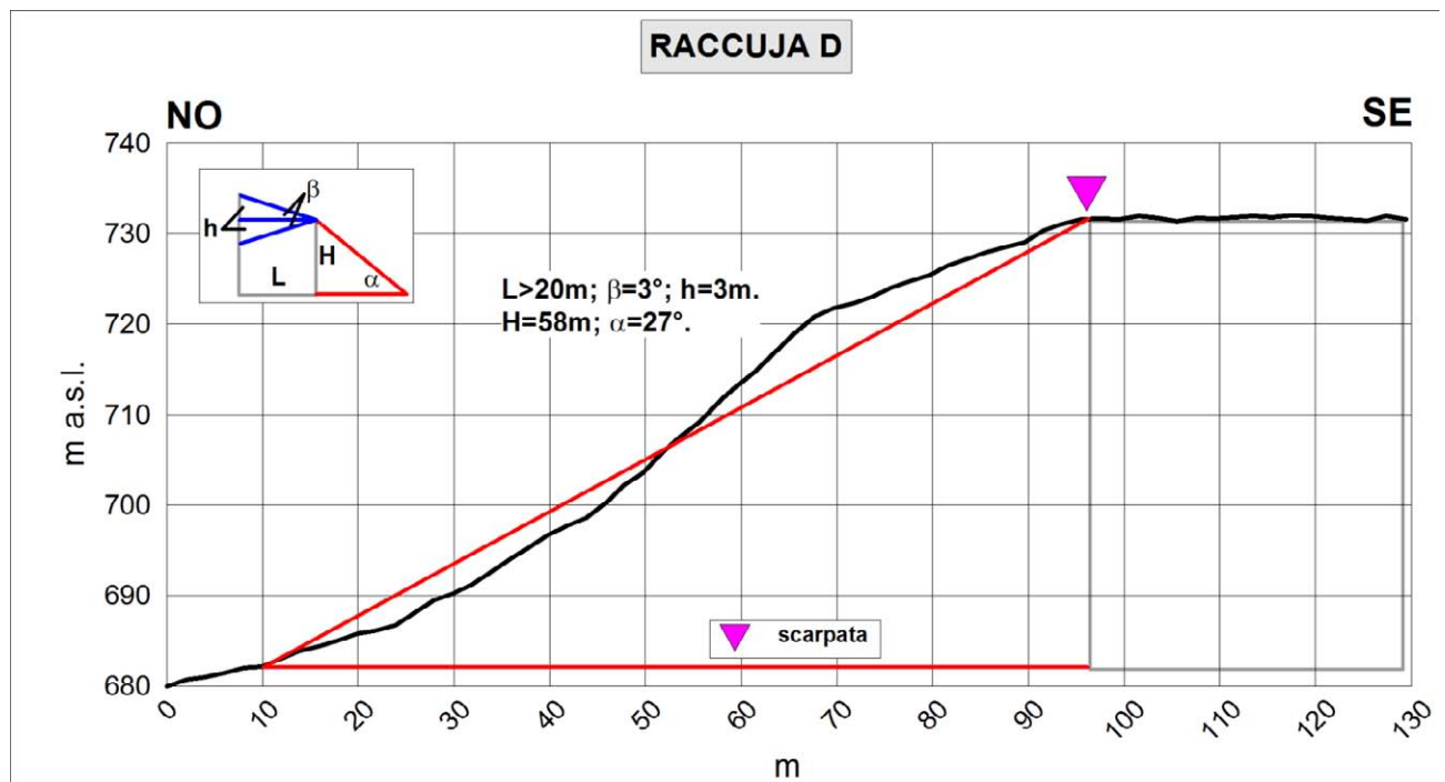
Fig. 8.20 – Profilo topografico di dettaglio della scarpata Raccuja D1.
