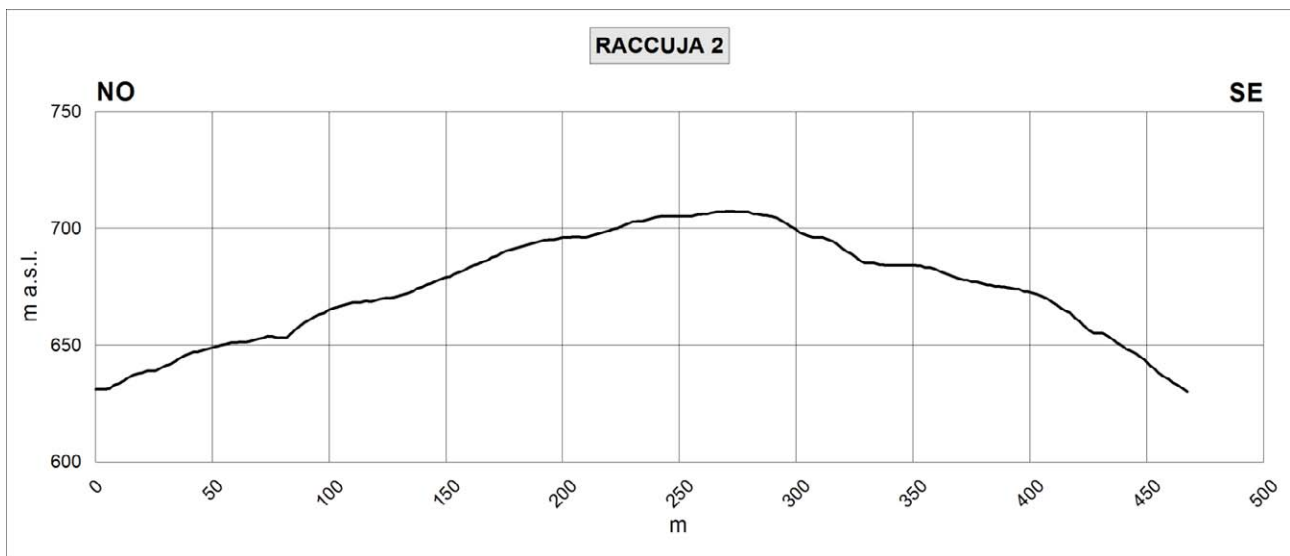
Fig. 3.8b – Profilo topografico di inquadramento Raccuja 2.
